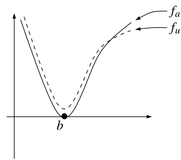
b ist Nullstelle höherer Ordnung von f_a
